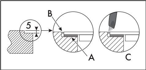
Нормально и заподлицо встраиваемый вариант (мм)*
