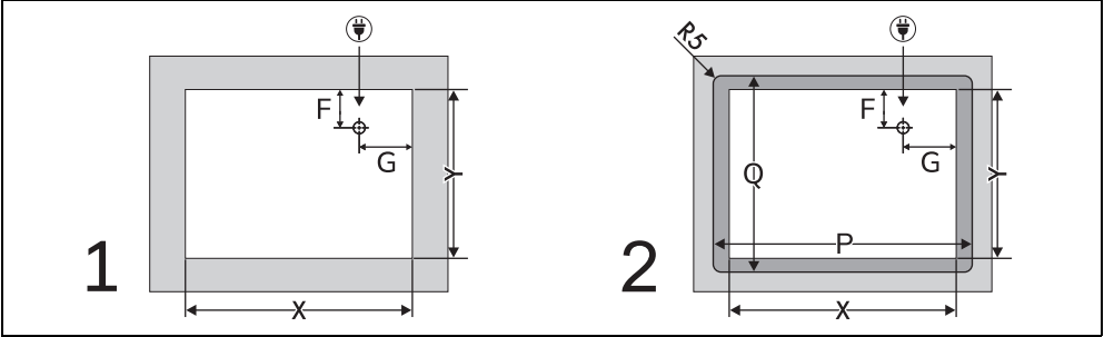
Нормально и заподлицо встраиваемый вариант (мм)*
